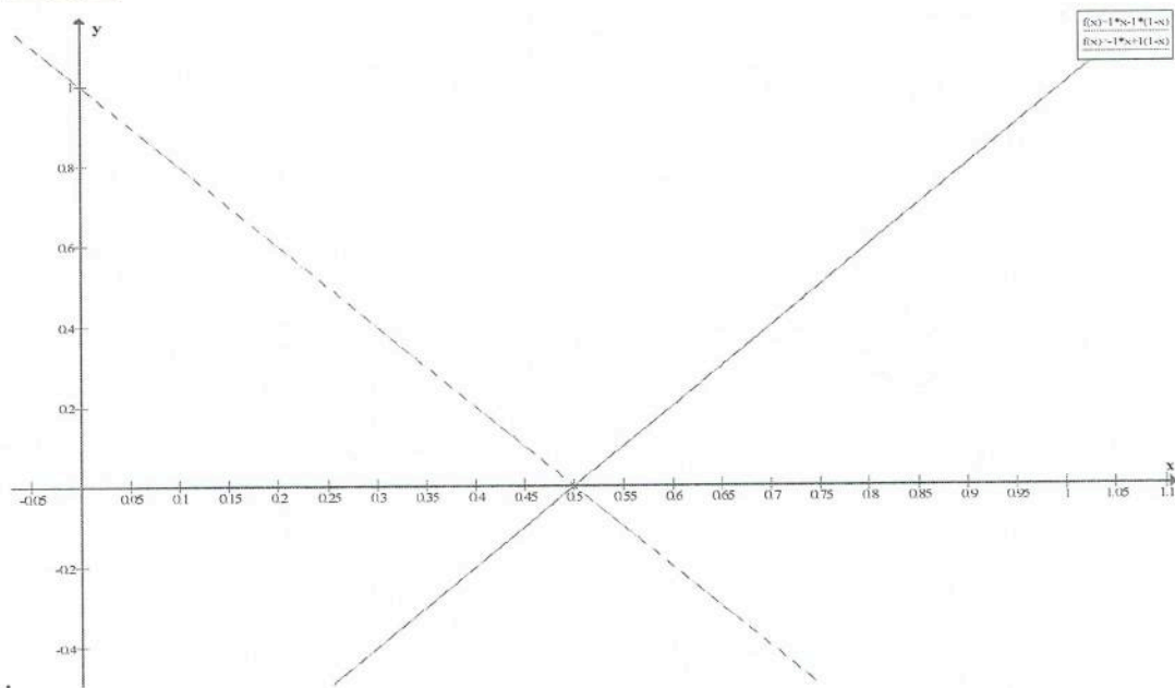
Figur 1 Dette er en geometrisk afbildning af udbyttefunktionerne for spiller A, i dette tilfælde er det den samme som for spiller B.
